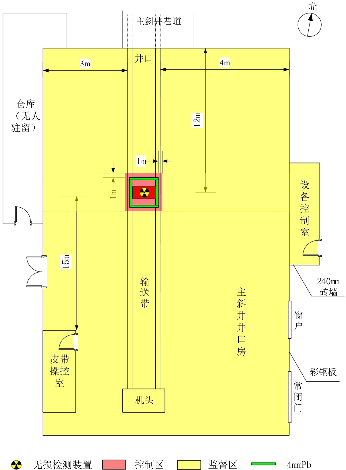
无损检测装置分区管理示意图
