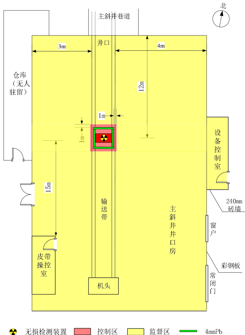
图 11-1 主斜井输送带无损检测装置分区管理示意图
